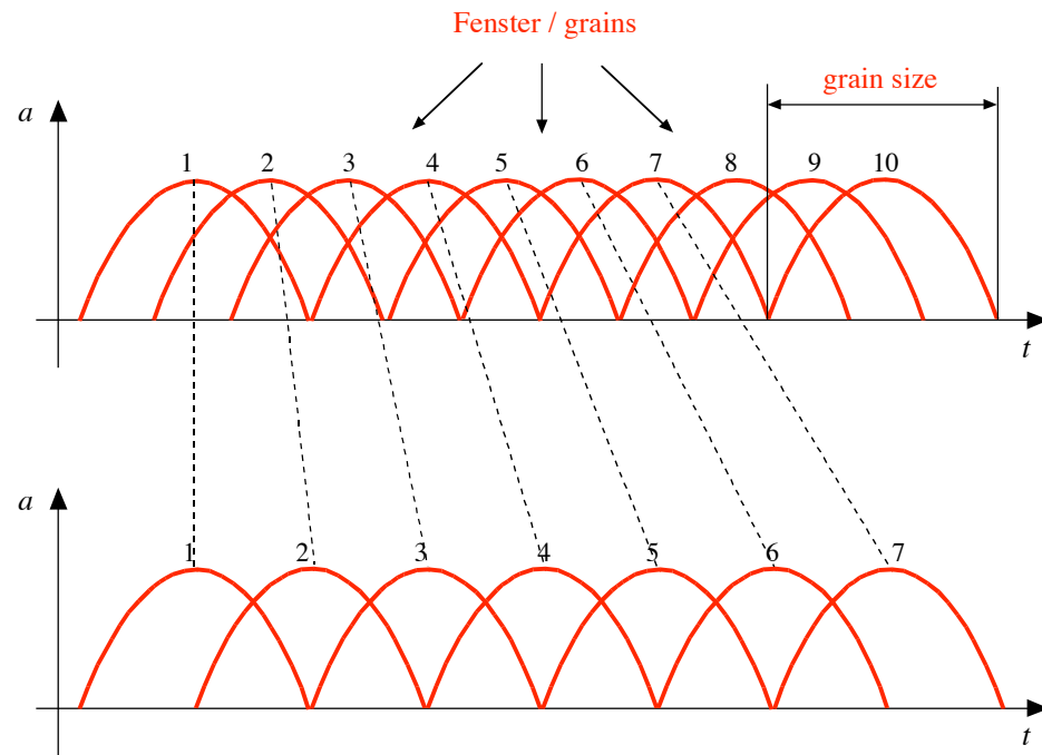
im Verhältnis 3:2 verlängertes Tonsignal
