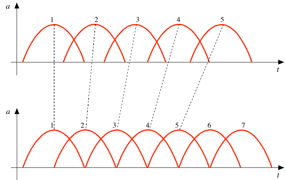
im Verhältnis 2:3 verkürztes Tonsignal
